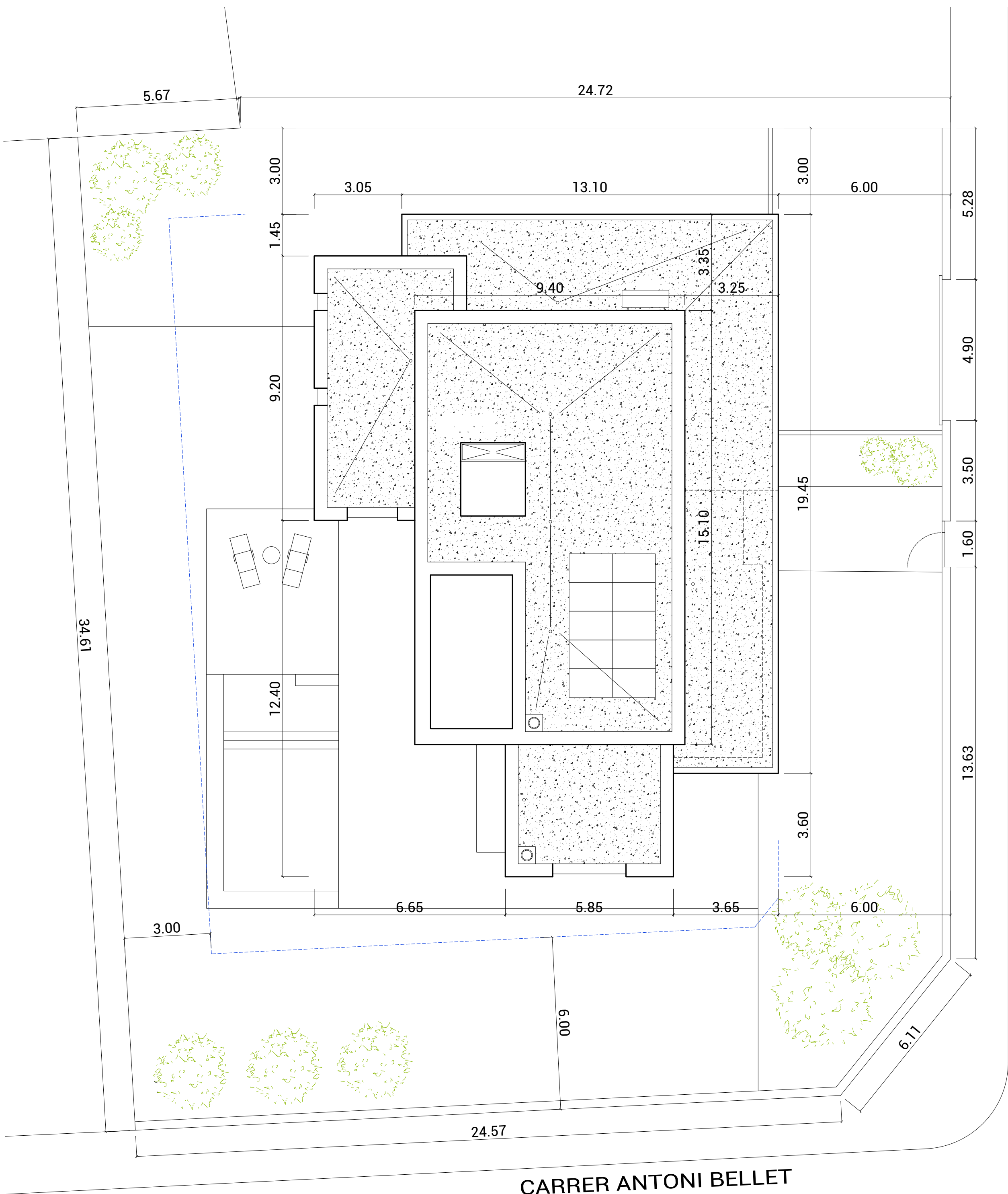
PLANTA COBERTA E. 1/100
