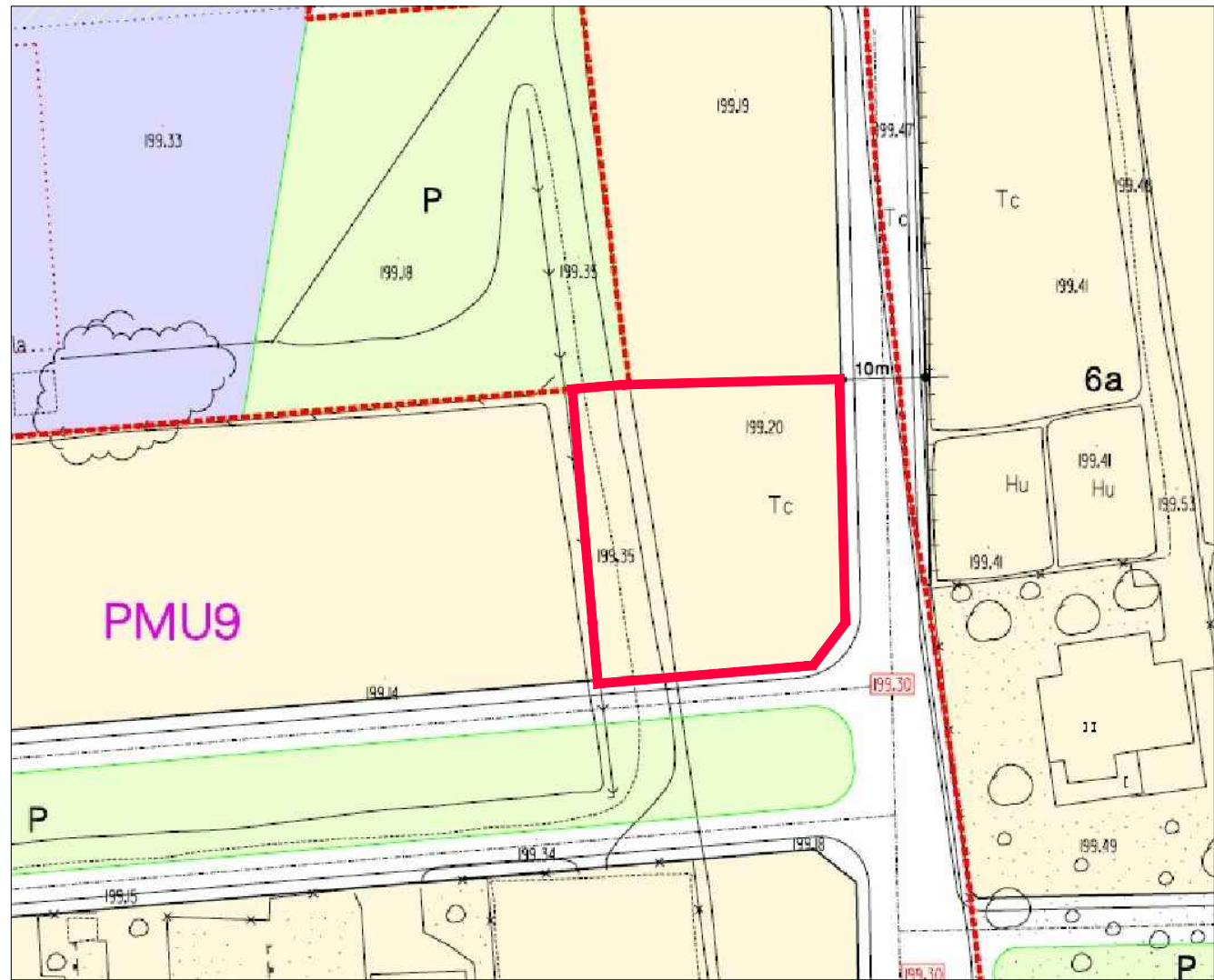
AEREA E. 1/750
